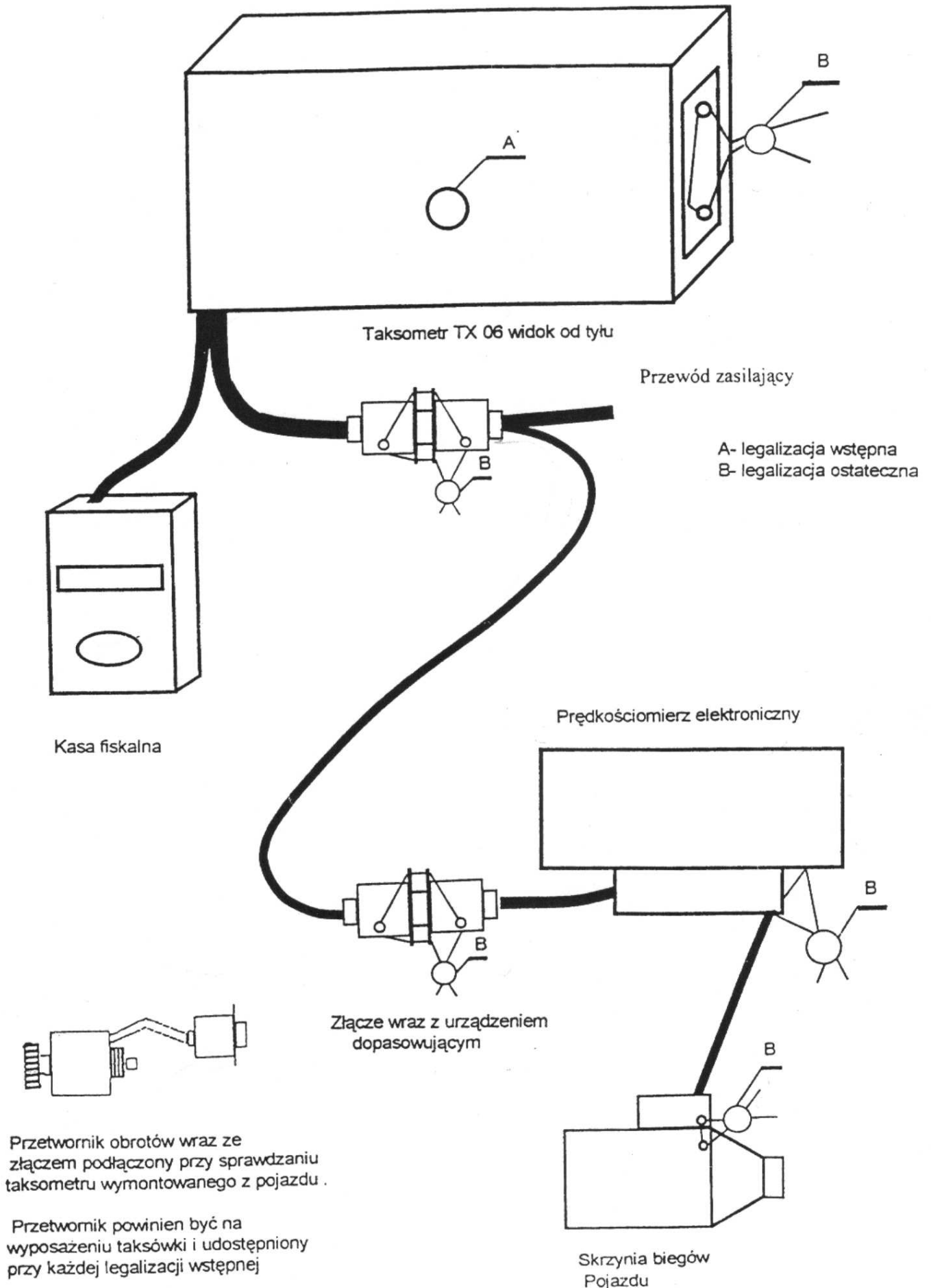
Rys. 2 Sposób zabezpieczeń taksometru sterowanego z układu częstotliwościowego elektronicznego prędkościomierza pojazdu
